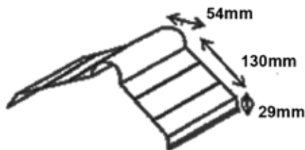
RollTopRidge
